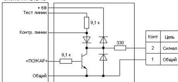
Схема ИП 212-43
